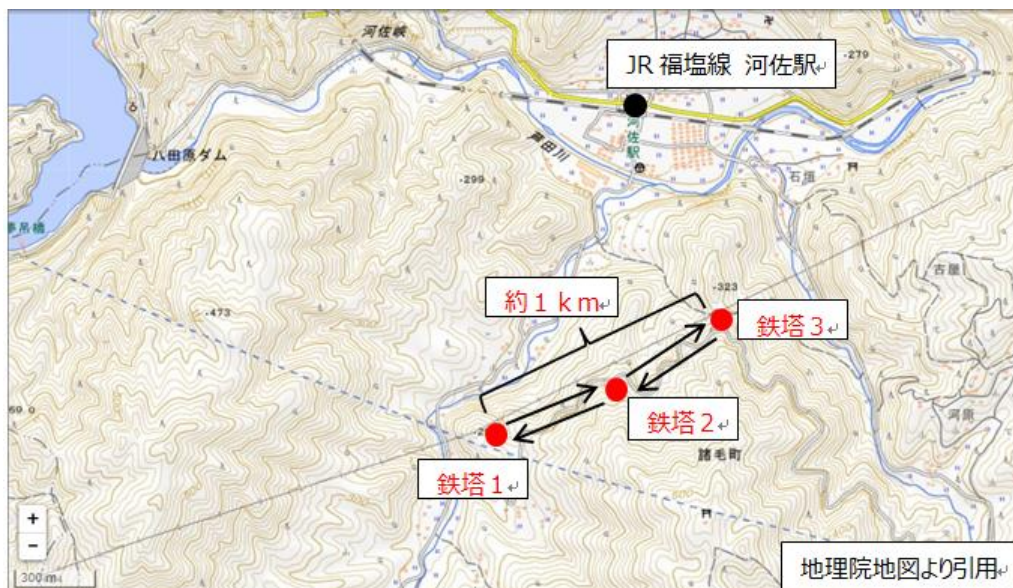
飛行経路図
